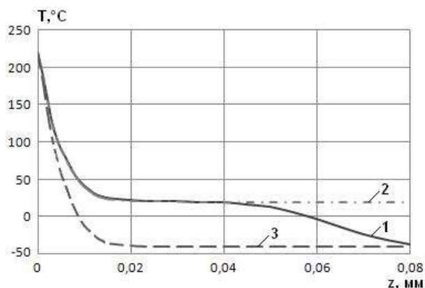
Рисунок 1 – Распределение температуры по длине трубы в момент завершения этапа нагрева, 1 – T_0 = 40^\circ\text{C} с подогревом, 2 – T_0 = 20^\circ\text{C} , 3 – T_0 = -40^\circ\text{C} без подогрева (название рисунка шрифт 12, выравнивание – по центру, интервал после – 6 пунктов)
